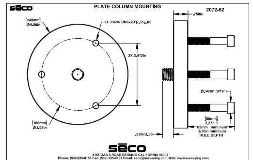
2072-52 — Column Plate
